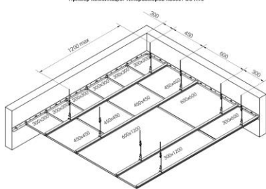
Пример комбинации типоразмеров кассет ЗС К190
