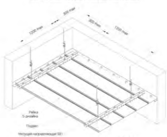
Стандартный монтаж реечного потолка французского S-дизайна
