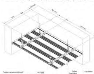
Монтаж на подвес с пружинный край реечного потолка французского S-дизайна
